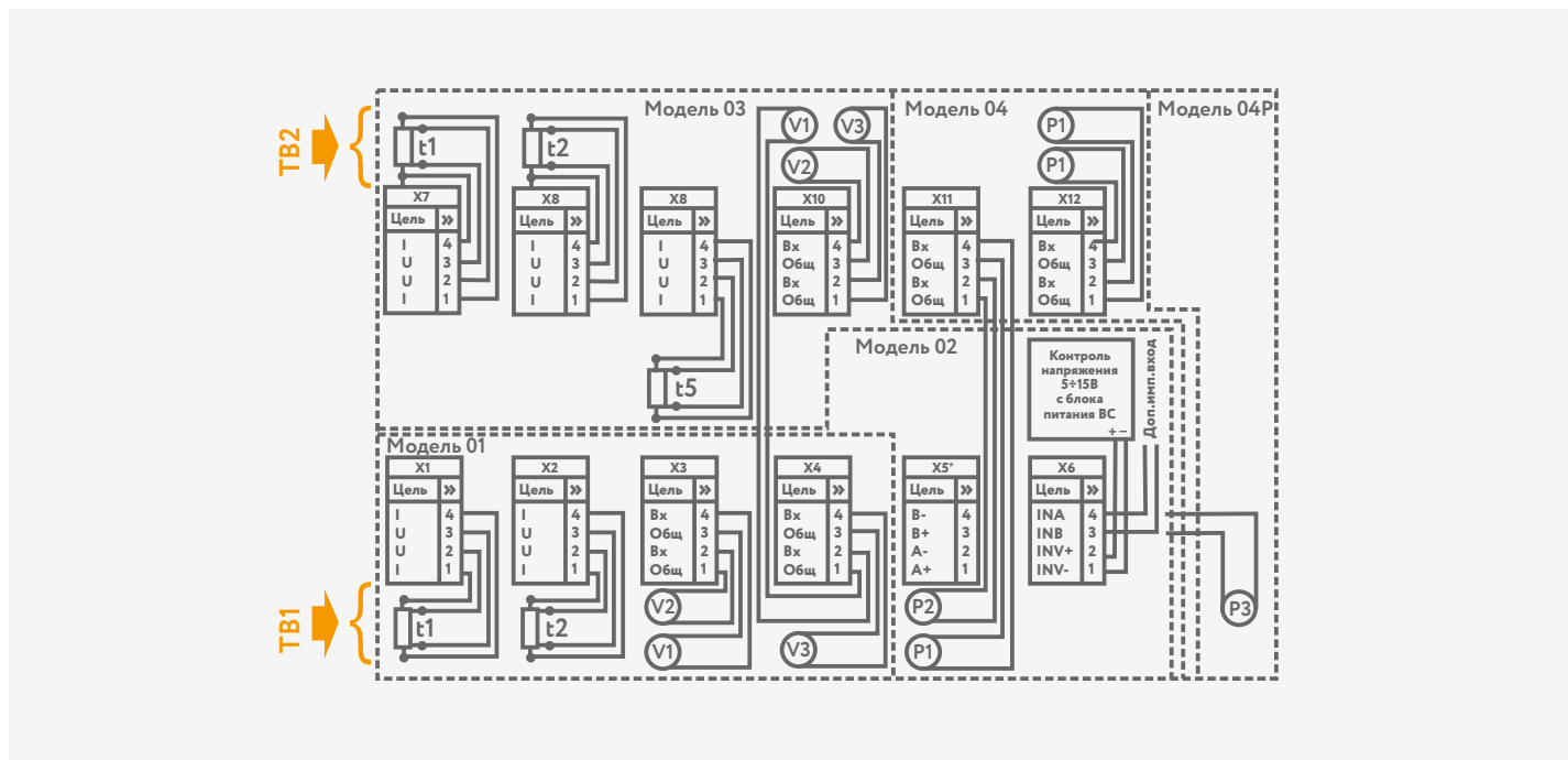
Рис. 5.4 Схема подключения датчиков к разъемам ВКТ-7
