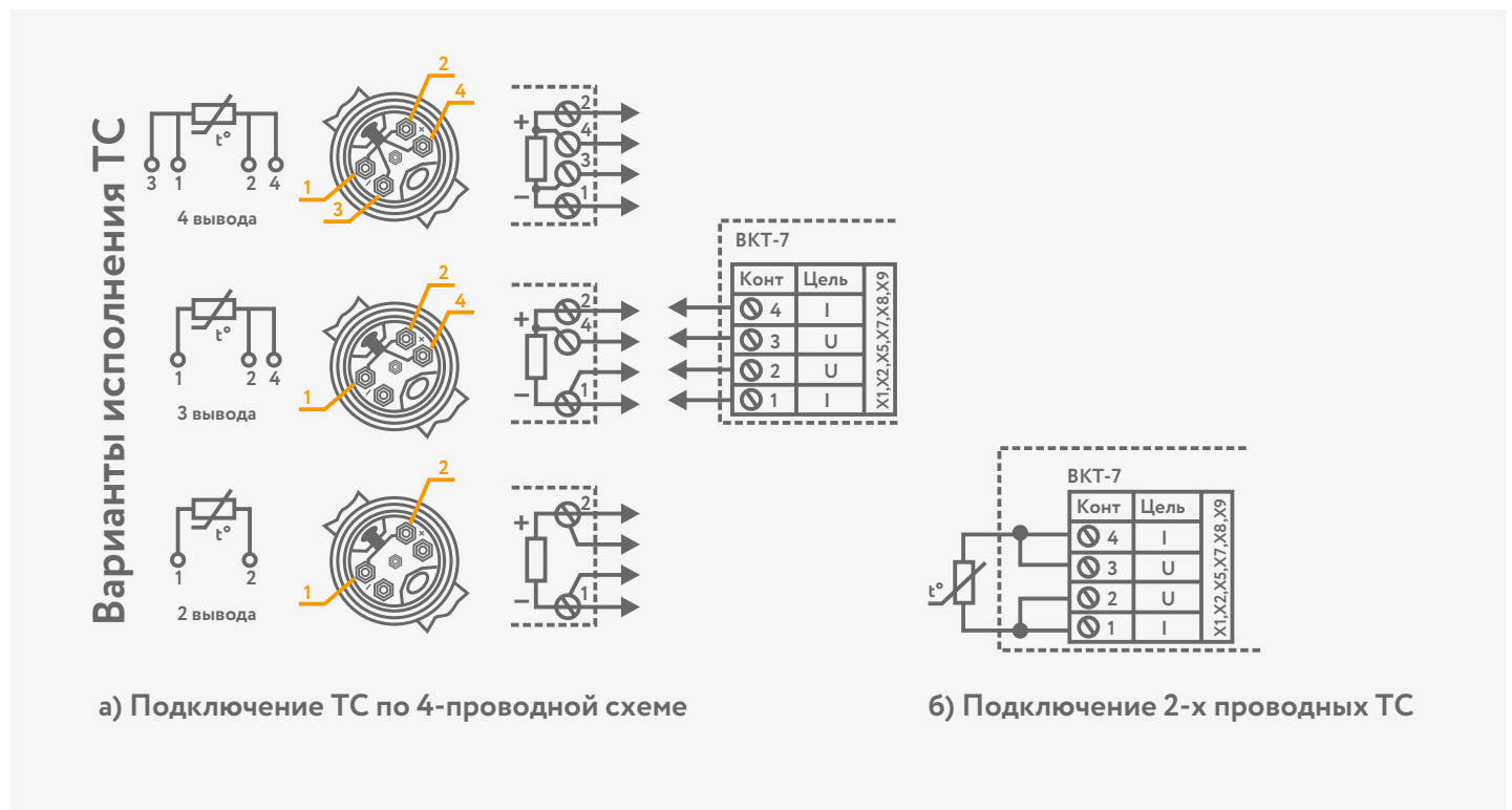
Рис. 5.2 Варианты подключения ТС
