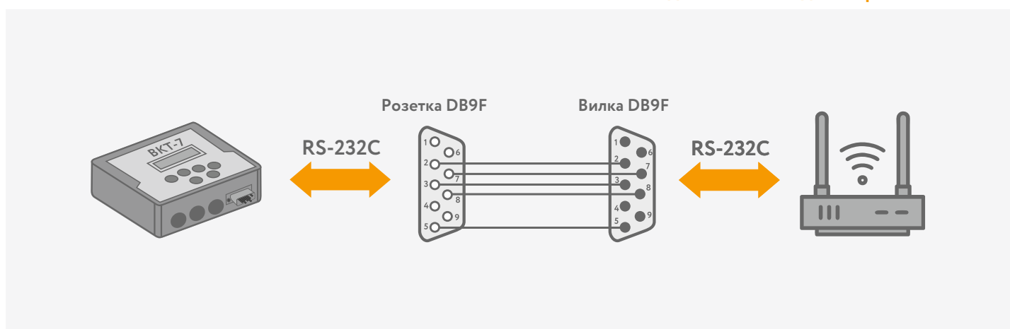
Схема подключения модема с разъемом DB9M
