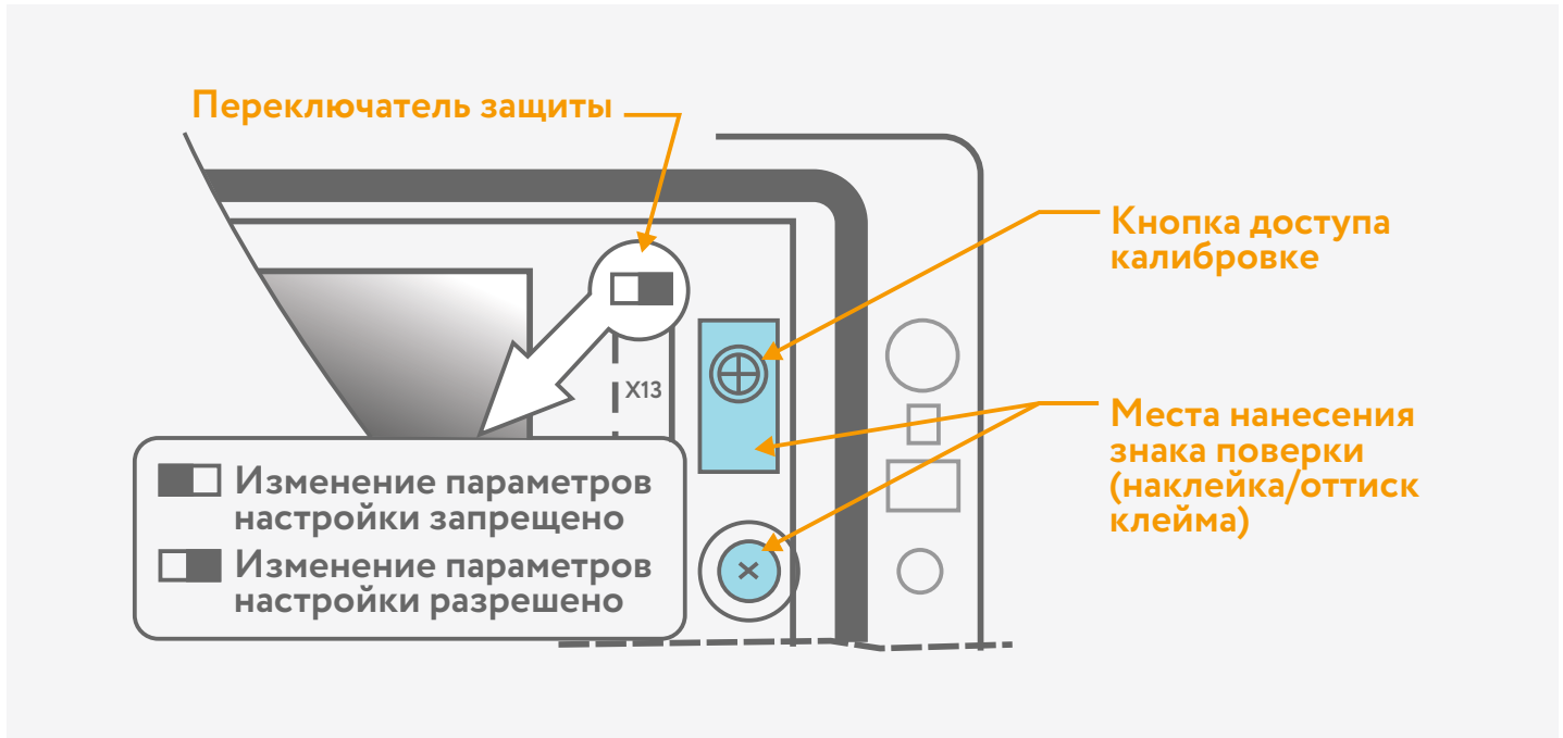
Рис. 1.2 – Места пломбирования поверителем
