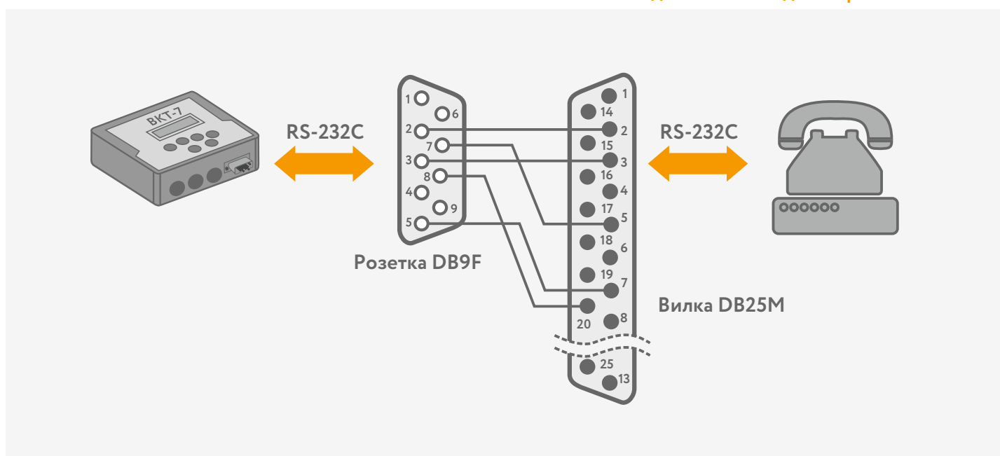
Схема подключения модема с разъемом DB25M
