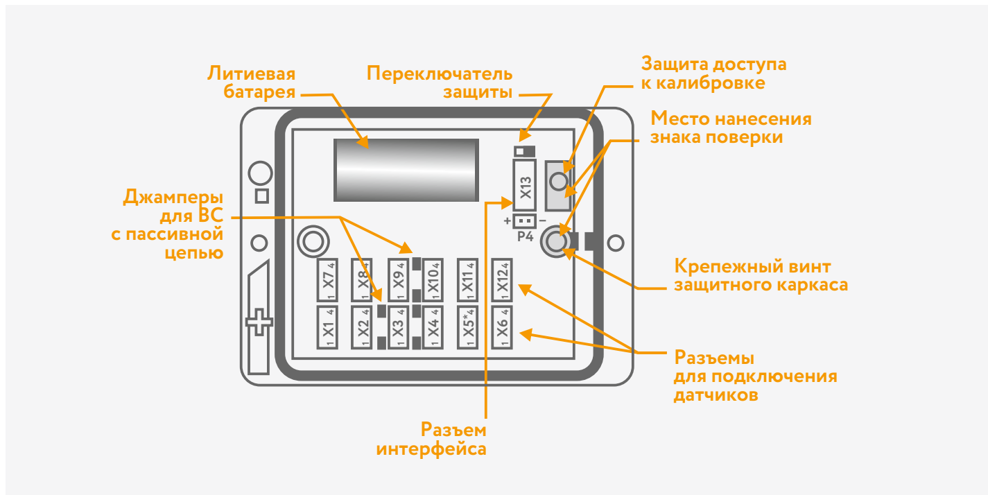
Рис. 5.3 Вид снизу на снятую крышку ВКТ-7
